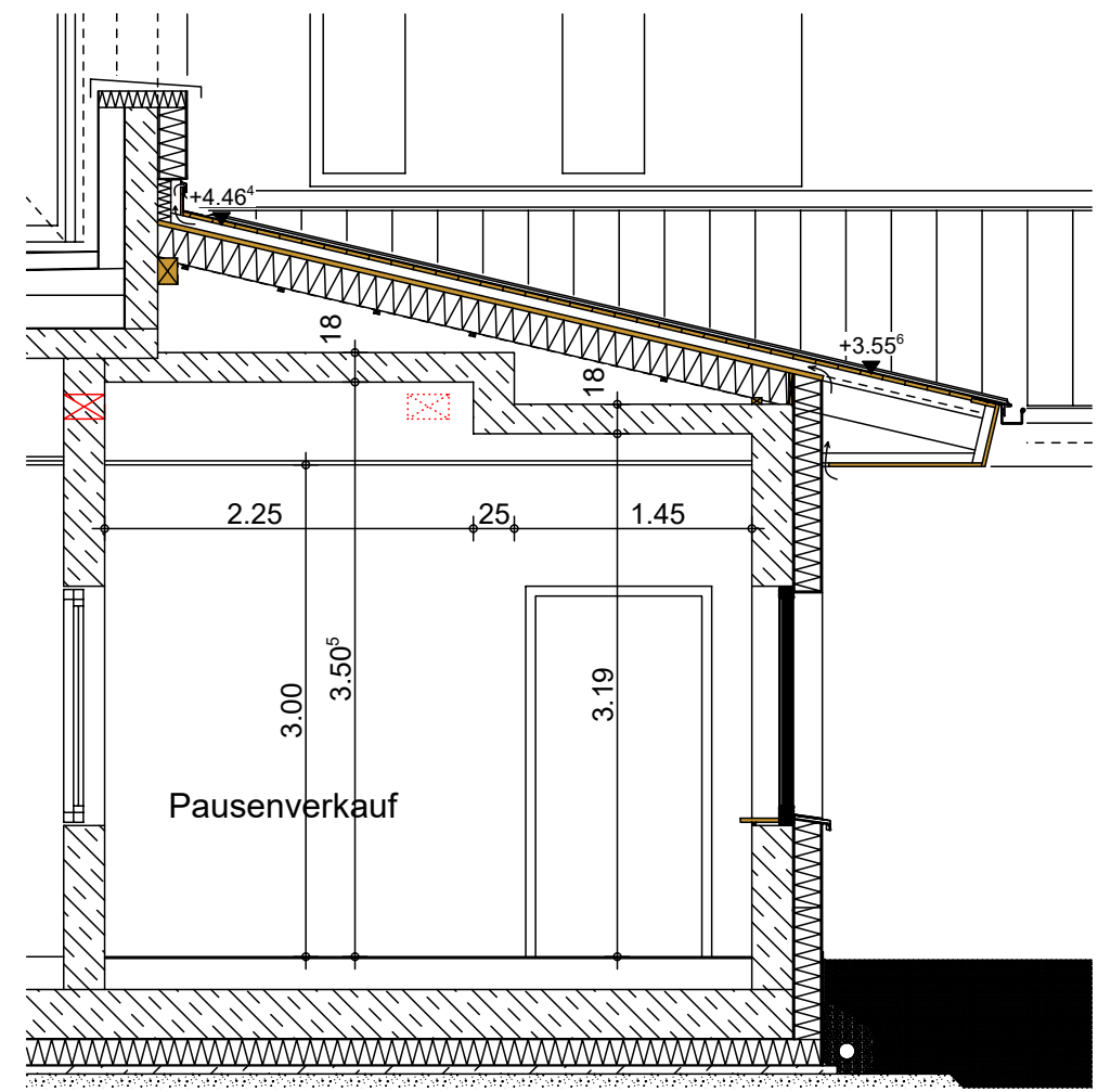
Schnitt A2
