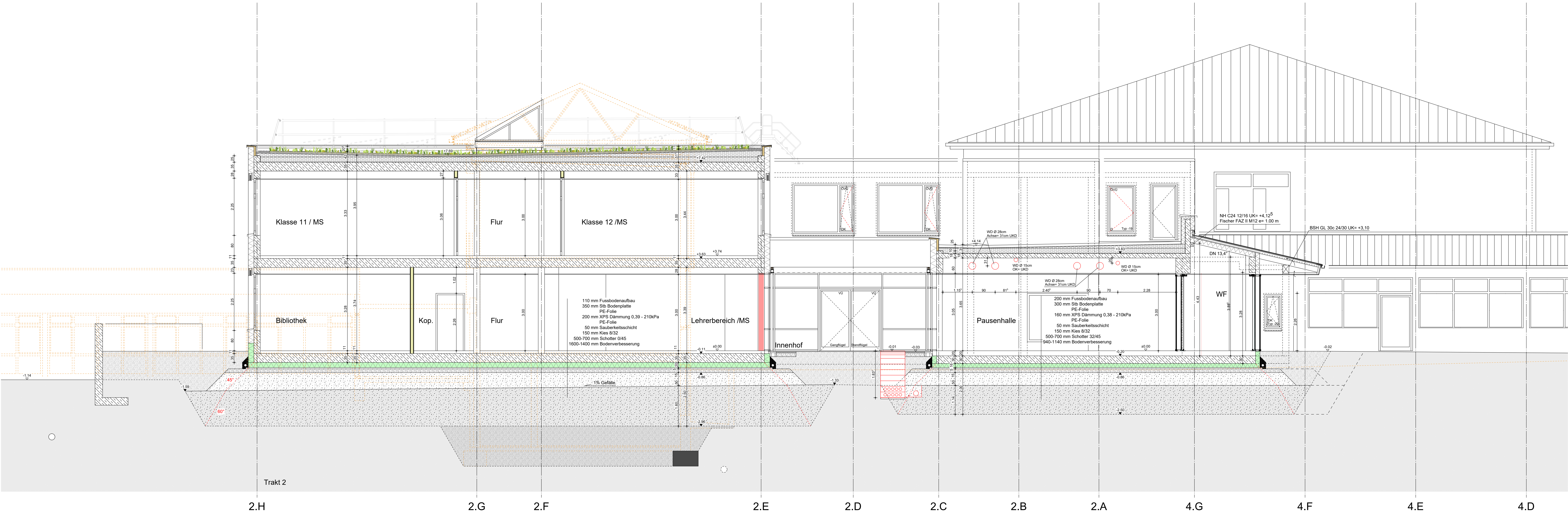
Schnitt A
