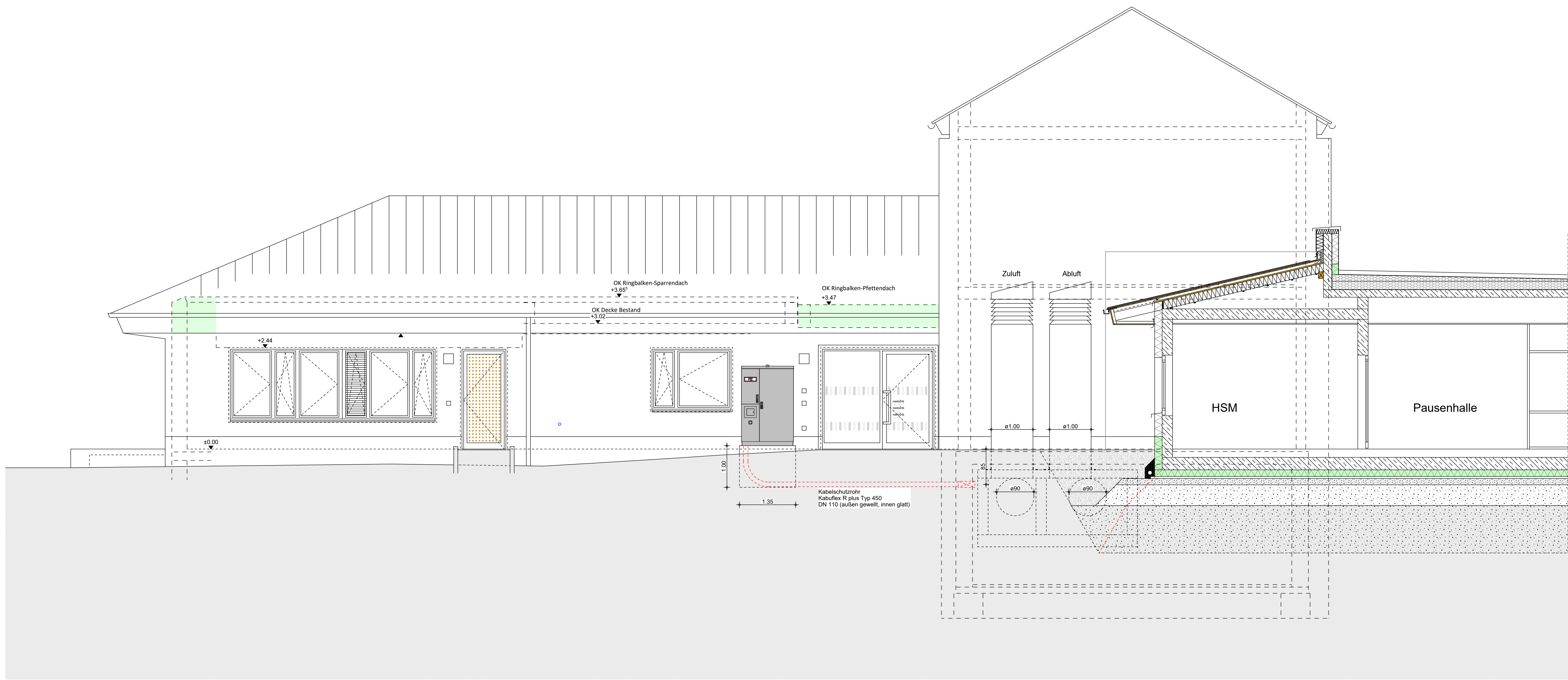
Schnitt A1
